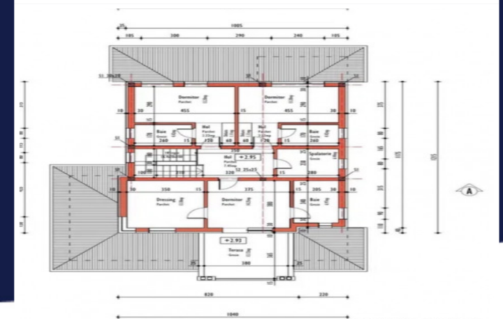
PLAN ETAJ SCARA 1:100
