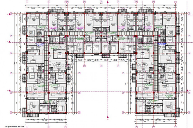
PLAN ETAJ II
